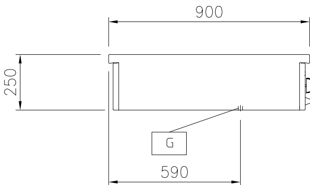
Zij aanzicht
